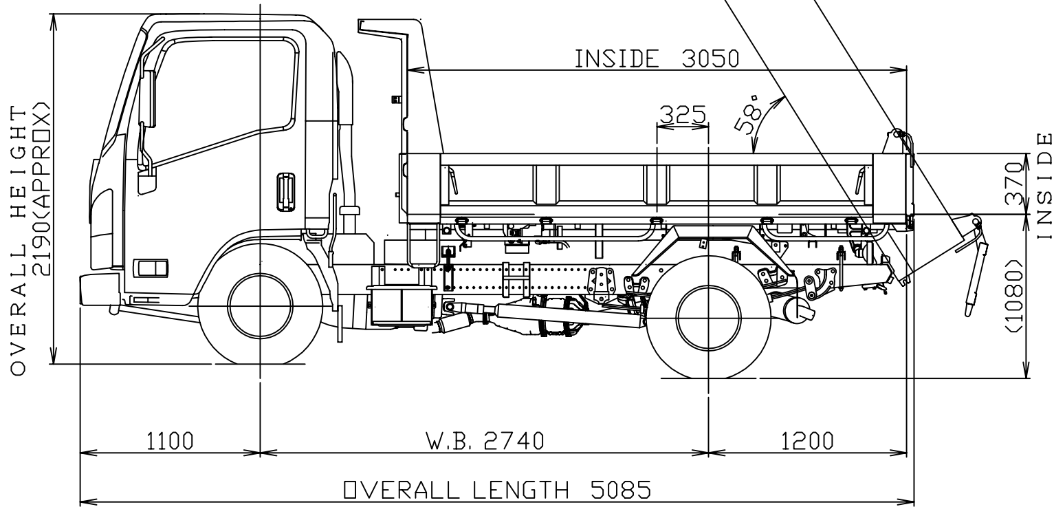
NH 2011MY Isuzu NLS 200 AWD tipper
